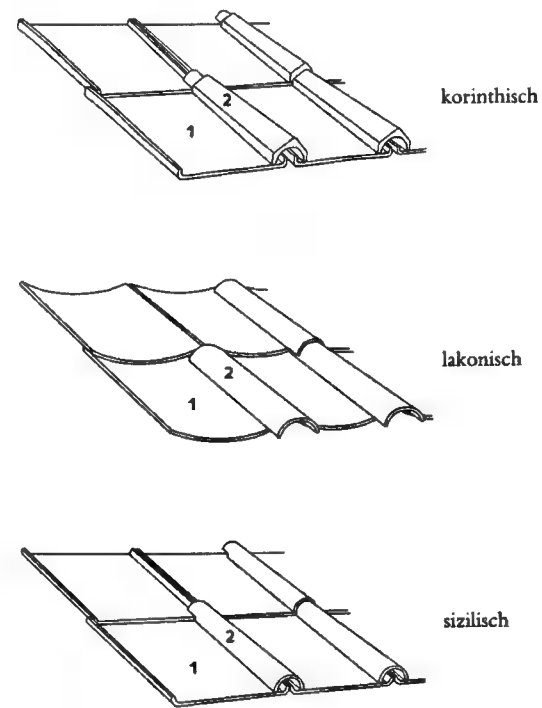
1 Ziegel 2 Kalyptrae Formen der Dachdeckung mit Ziegeln
